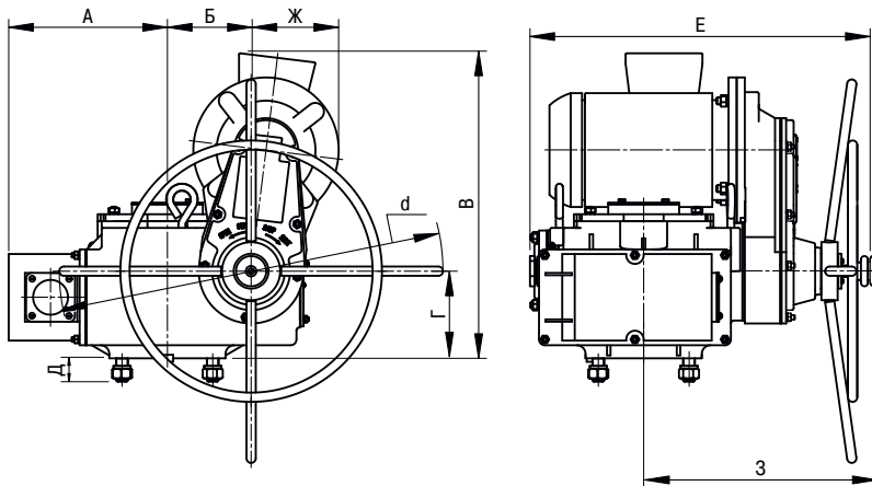
Взрывозащищенное исполнение
