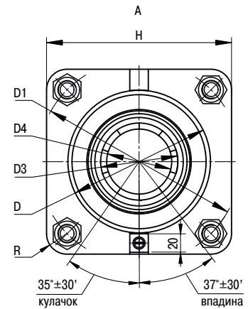
Присоединительные размеры
